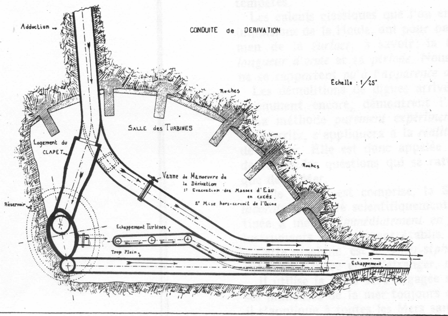
Plan de l'étage des turbines. Détail des conduites, système de dérivation. (Plan d'exécution.) (Figure 5.)
