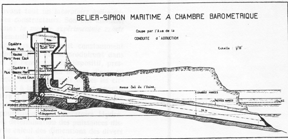
Coupe par l'axe de la conduite d'adduction. (Plan d'exécution.) (Figure 4.)
