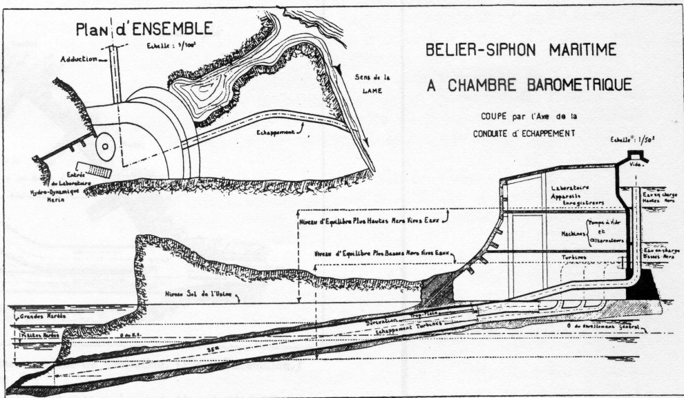
Plan d'ensemble et coupe par l'axe du collecteur d'échappements. (Plans d'exécution.) (Figure 3.)
